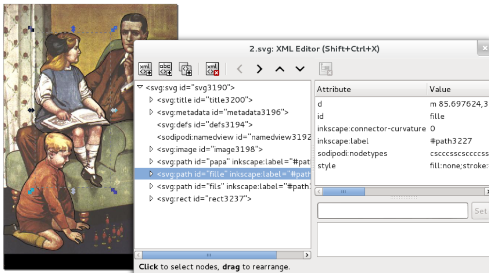
FIGURE 10 – L'éditeur XML d'Inkscape permet de contrôler l'ordre d'affichage des détails dans l'image interactive. Remarquez la mise en évidence d'un élément sur l'image de fond par simple sélection dans l'éditeur.
