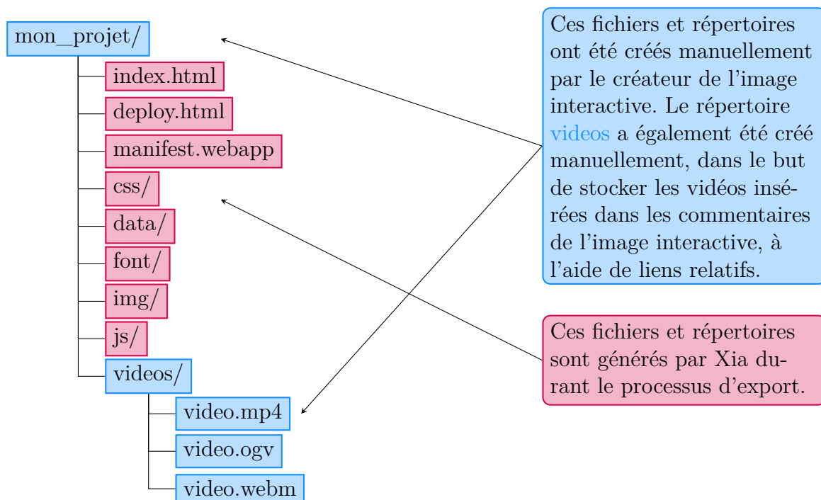
FIGURE 5 – Fichiers d'une image interactive avec l'export Firefox OS activé
