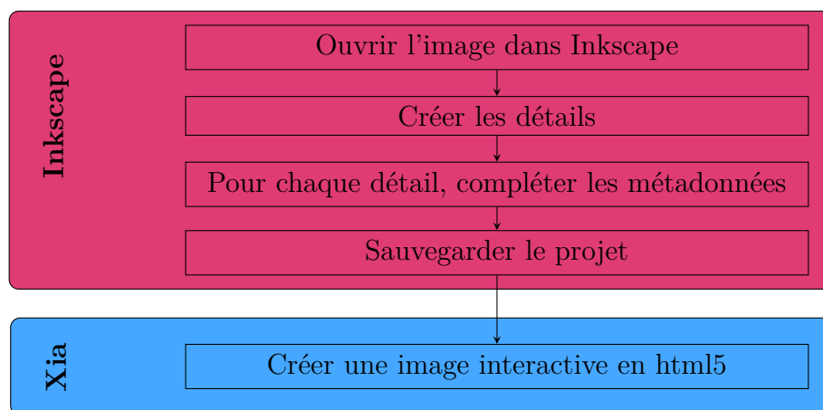
FIGURE 1 – Processus de création d'une image interactive avec Xia
